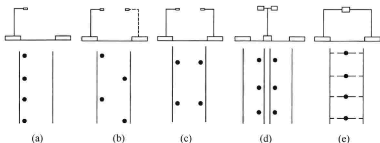
图 5.1.3 常规照明灯具布置的五种基本方式
